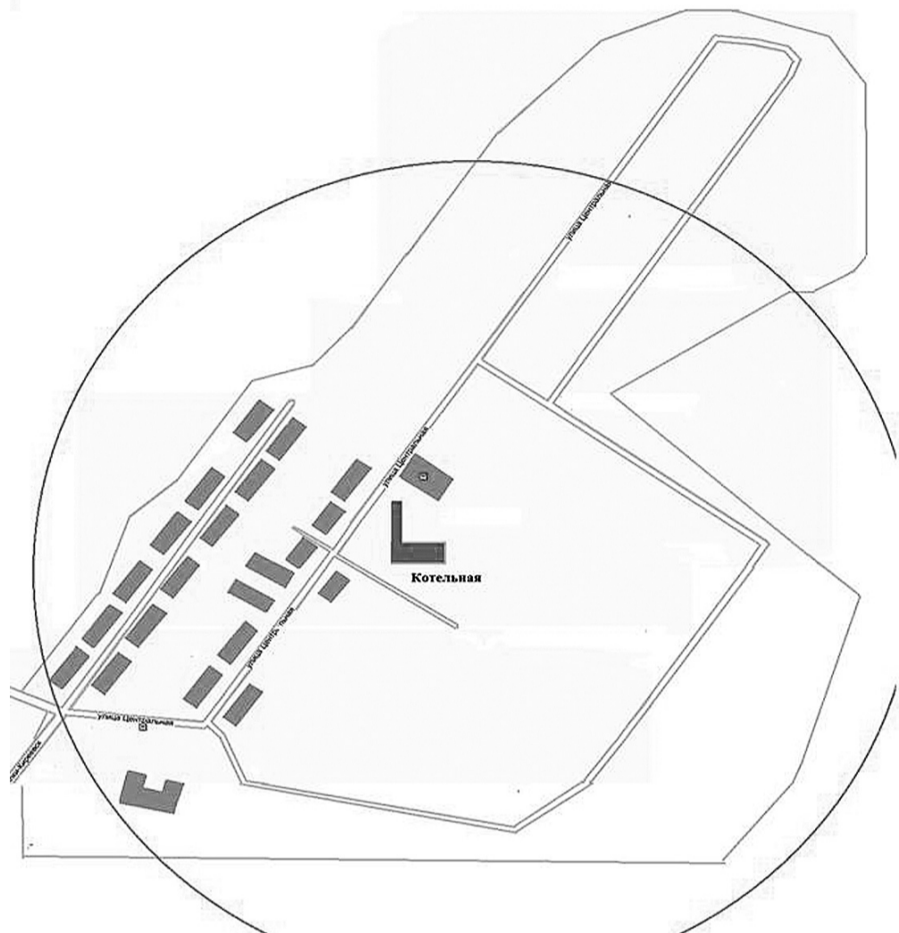
Рисунок 3.4.1. Радиус эффективного теплоснабжения п. Ломинцевский.
