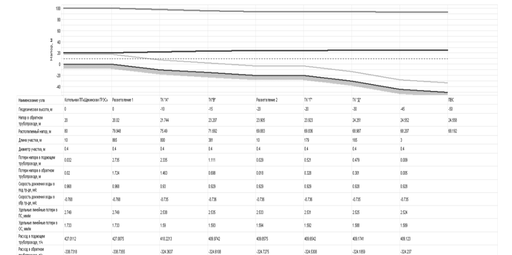
Рис. 7.2. Пьезометрический график магистральных трубопроводов от ООО «Щекинский ГРЭС» до ПНС при температурном графике работы 130-70 °С. Удельными линейными потерями напора не превышающими нормативные значения
