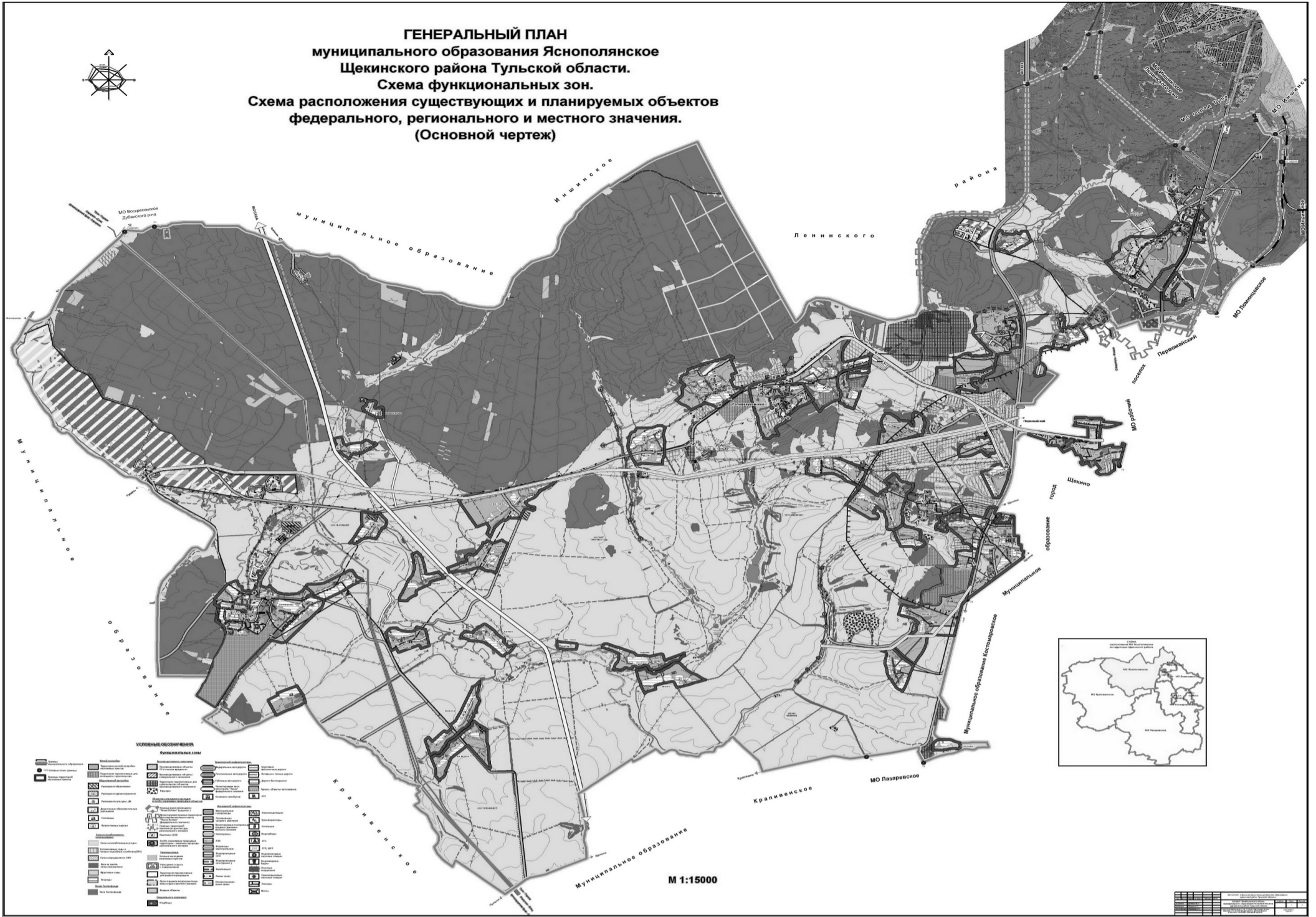
Фрагмент ОСНОВНОГО ЧЕРТЕЖА генерального плана МО Яснополянское (д. Б. Тросна - исходный вариант)
