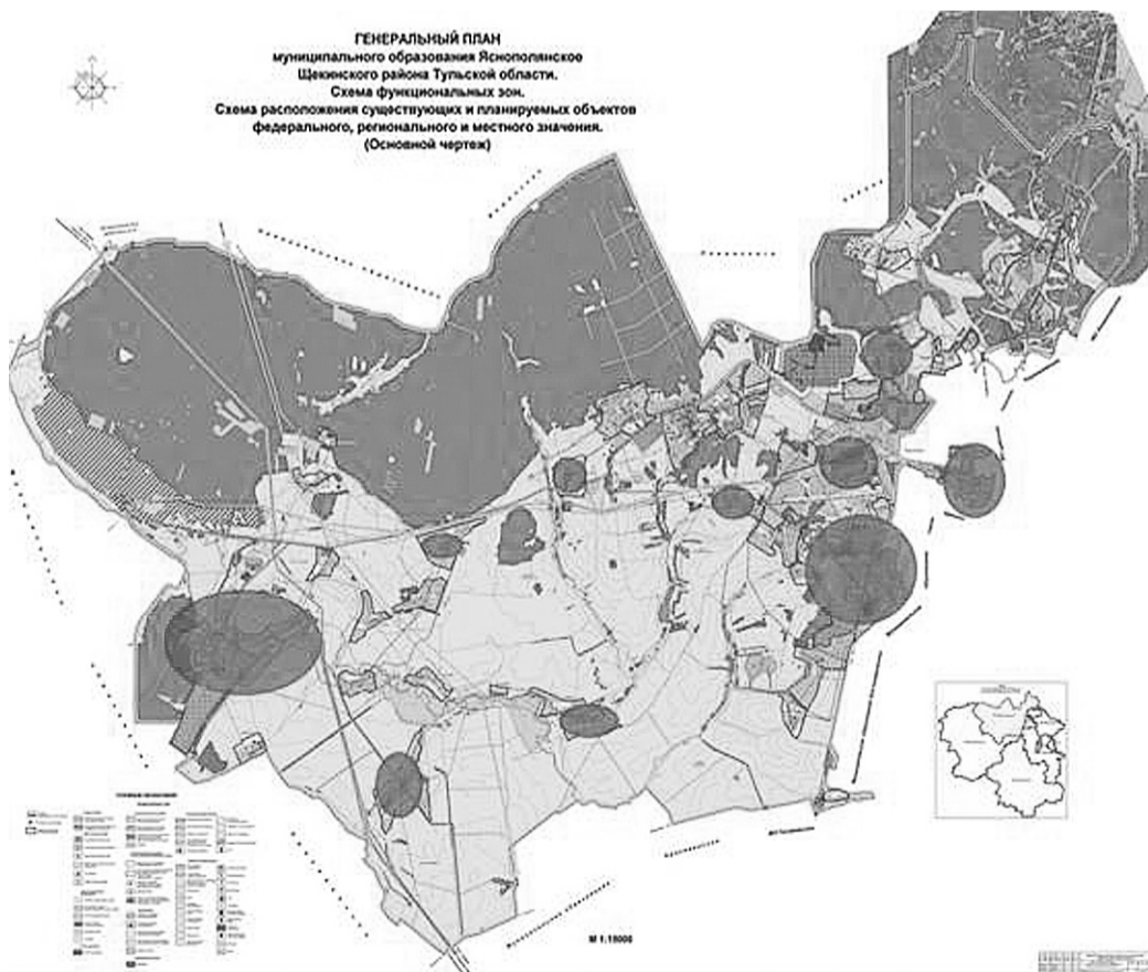
Зоны, неохваченные системой централизованного водоотведения
