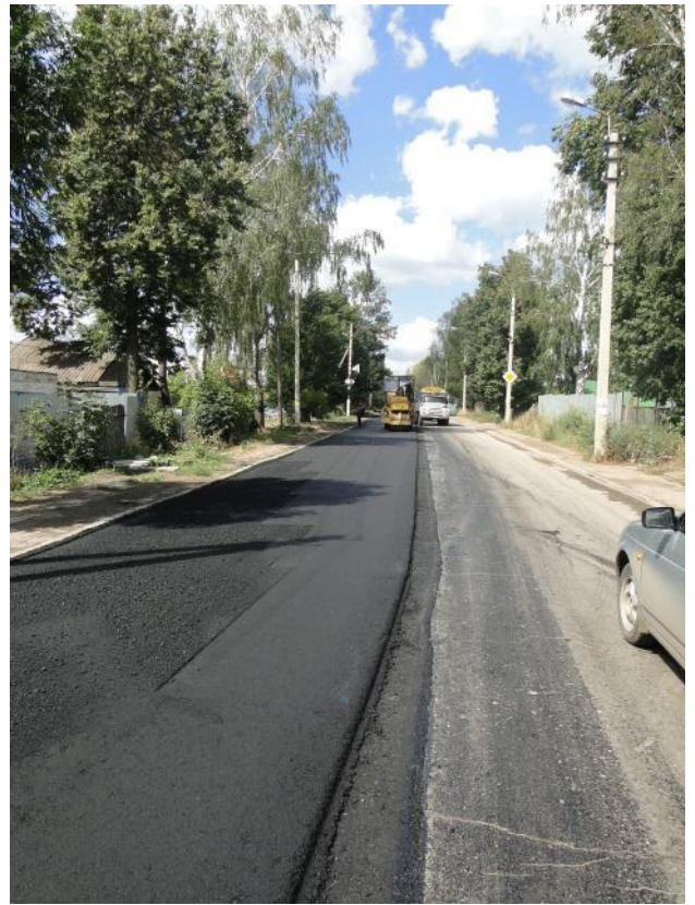
Укладка асфальта
