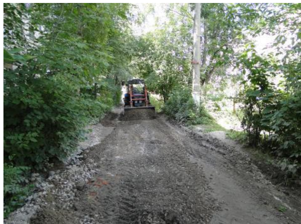
д.6 Выравнивание поверхности
