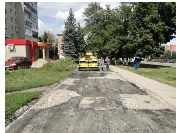
Устройство выравнивающего слоя
